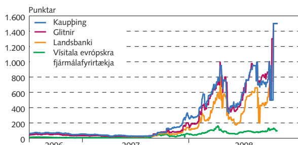
Skuldatryggingar íslenskra banka og vísitala evrópskra fjármálafyrirtækja Daglegar tölur 8. júlí 2006 - 16. október 2008
