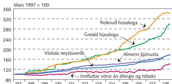
I-11 Verðlagsþróun Vörur, húsnæði og þjónusta
