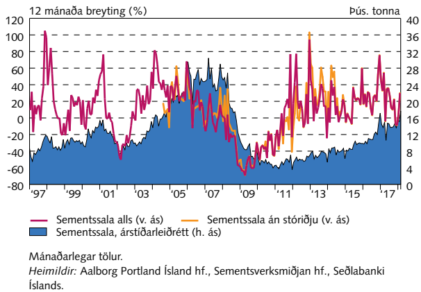
Sementssala
